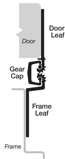
Fig. 3 Door Open 180°
